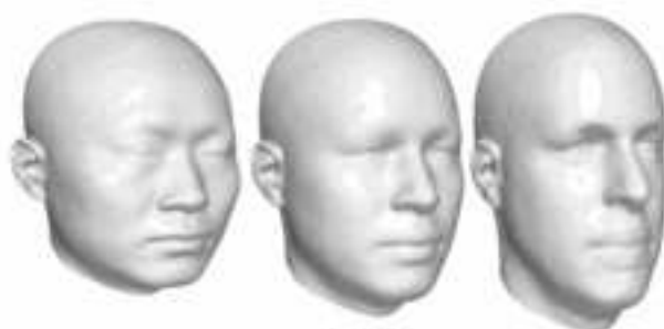
PC2
