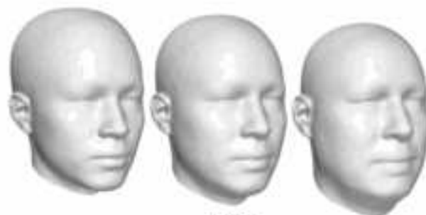
PC5
