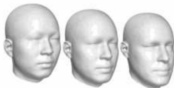
PC3
