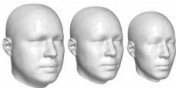
PC1
